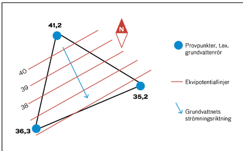
Figur 1 Grundvattnets strömningsriktning kan bestämmas med en så kallad "hydraulisk triangel" där nivåerna mäts i tre punkter. Strömningsriktningen (den blå pilen) ligger vinkelrätt mot ekvipotentiallinjerna (de röda linjerna).
