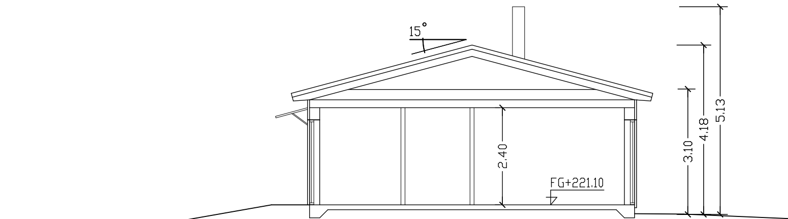
SEKTION A - A
