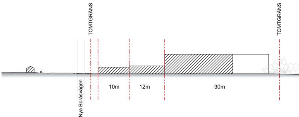
Sektion inom en del av planområdet som visar hur bebyggelsen trappas upp. Se situationsplanen nedan för vilket område sektionen avser. Bsv arkitekter & ingenjörer ab, 2023.
