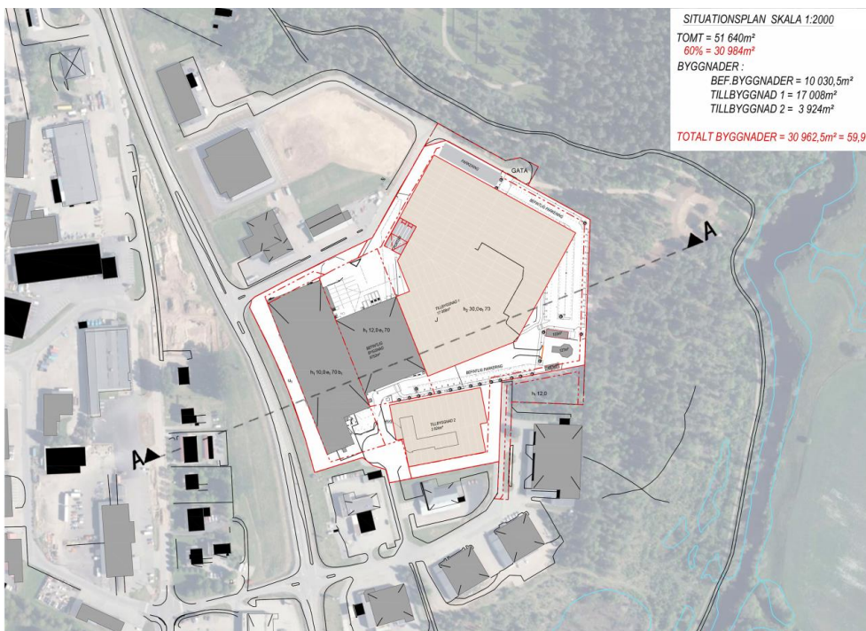
Situationsplan som visar ett exempel på hur planområdet kan bebyggas. Situationsplanen redovisar även vilket område sektionen i bilden ovan avser. Bsv arkitekter & ingenjörer ab, 2023.
