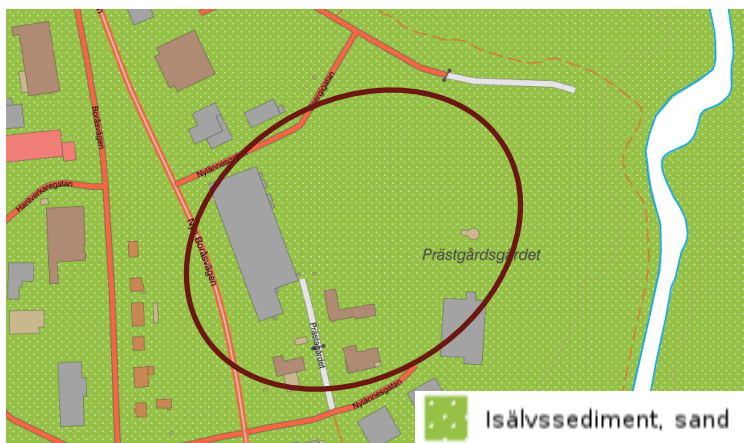
Karta hämtad från SGU som visar att jordarten inom planområdet utgörs av isälvs sediment, sand.
