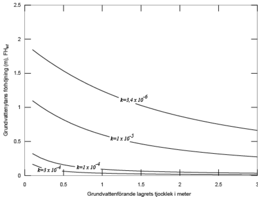
Figur 5 Grundvattennivåns förhöjning ( FH_{inf} ) som funktion av grundvattenförande lagrets tjocklek vid några olika k -värden. Kurvorna är beräknade baserat på metod beskriven av Finnemore 1993.
