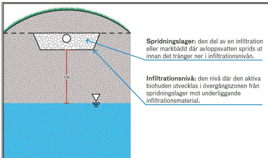
Figur 1 För att reningen i en infiltrationsanläggning ska fungera ska avståndet mellan infiltrationsnivån och den högsta dimensionerande grundvattennivån (den omättade zonen) vara minst 1 meter under större delen av året.
