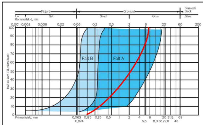
Figur 3 Siktanalys som visar att jordarten på platsen för infiltrationen ligger i fält A, vilket innebär att tillägg för höjning under infiltrationen inte behöver göras. FH_{inf}=0 .
