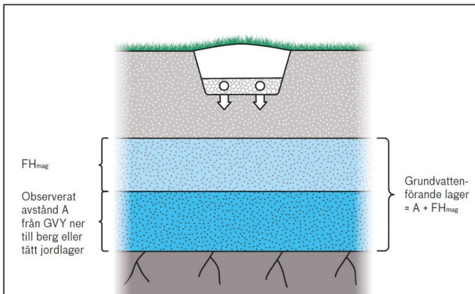
Figur 4 Principskiss över grundvattenförande lager. Har man räknat fram en korrigerad nivå för FH_{mag} så kan beräkningen av grundvattenförande lager beskrivas som denna nivå minus jorddjupet/avstånd till tät jordlager.
